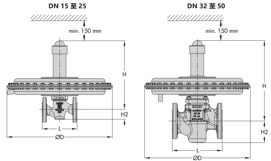
尺寸图
