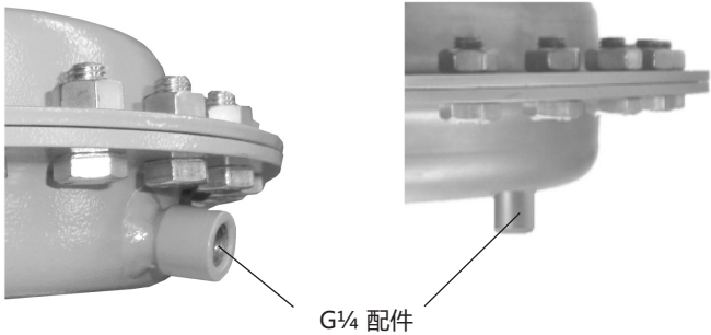
执行机构外壳侧面的导压管接头
