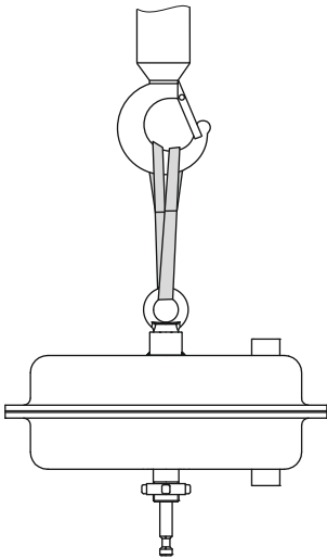
Bild 4-5: Hebepunkt am Antrieb
