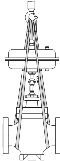
Bild 4-6: Hebepunkte am Stellventil (Beispiel)
