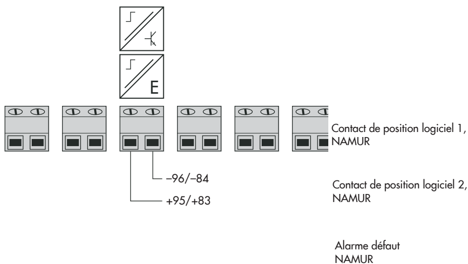
Affectation des bornes de la sortie binaire (sortie de l'alarme des défauts, NAMUR) et contact de position logiciel (NAMUR) – Option C
