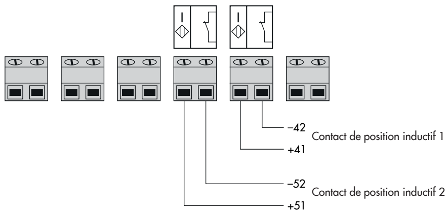
Affectation des bornes des contacts de position inductif – Option C
