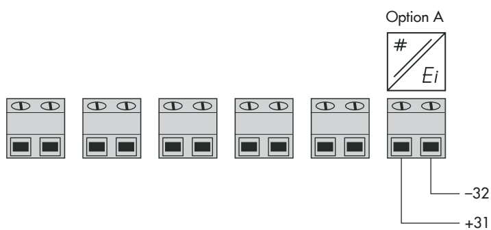
Affectation des bornes de la recopie de position – Option A
