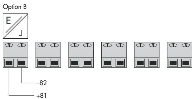
Affectation des bornes de la purge forcée – Option B
