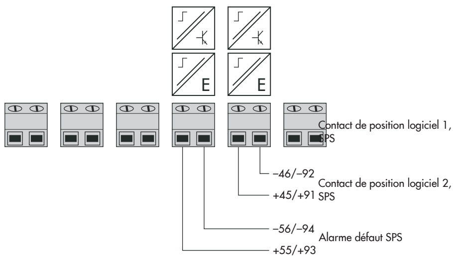
Affectation des bornes de la sortie binaire (sortie de l'alarme des défauts, SPS) et contact de position logiciel (SPS) – Option C
