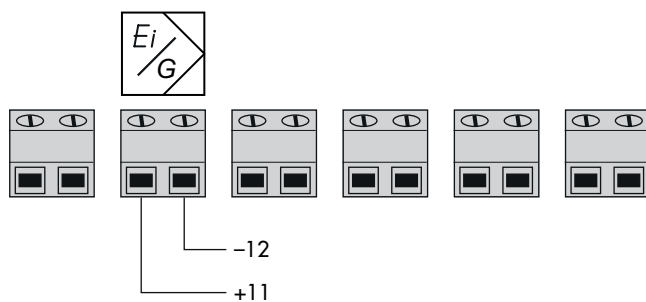
Raccord du signal de réglage en mA
