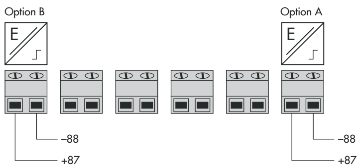
Affectation des bornes de l'entrée binaire – Option A/B
